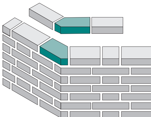
Mauerecke mit Formziegel D2
