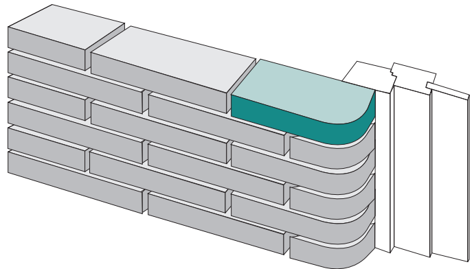
Fensterlaibung mit Formziegel B1
