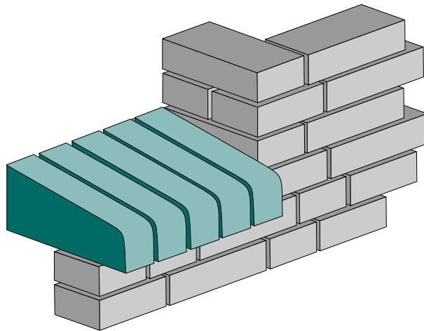
Sohlbank mit Formziegeln
